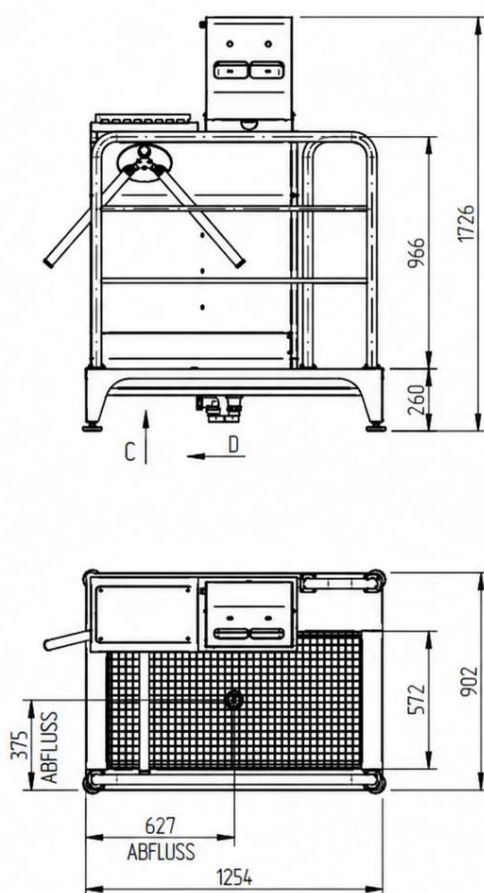
1227101020 DSO 01B.1P.1250
